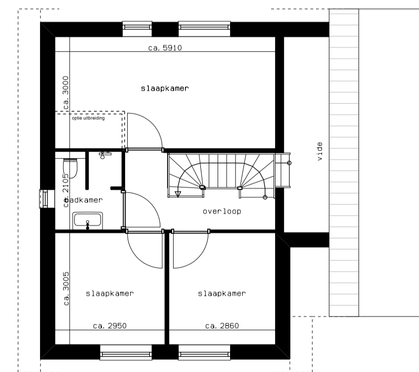
VERDIEPING 2.900+P
