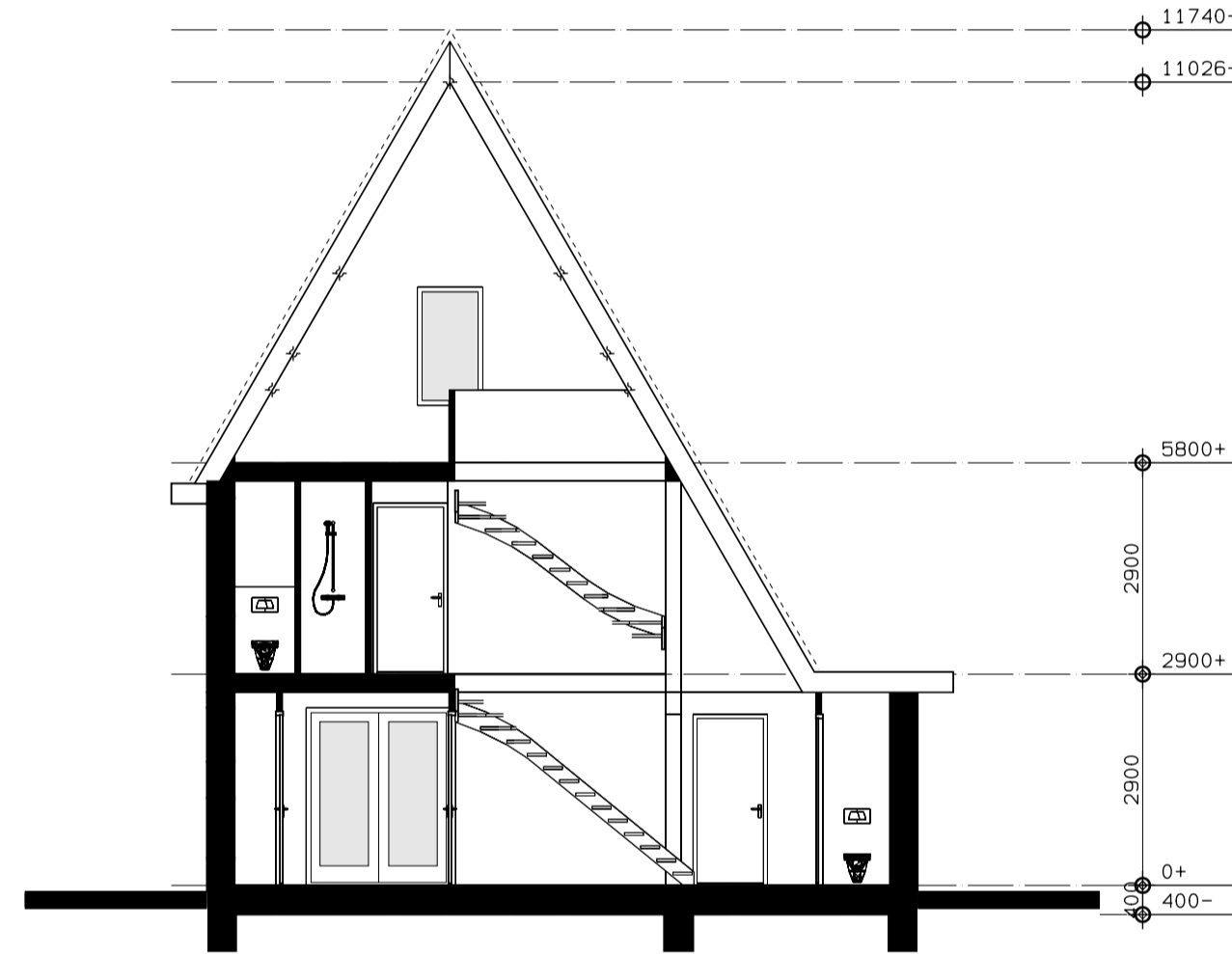
sneede A-A
