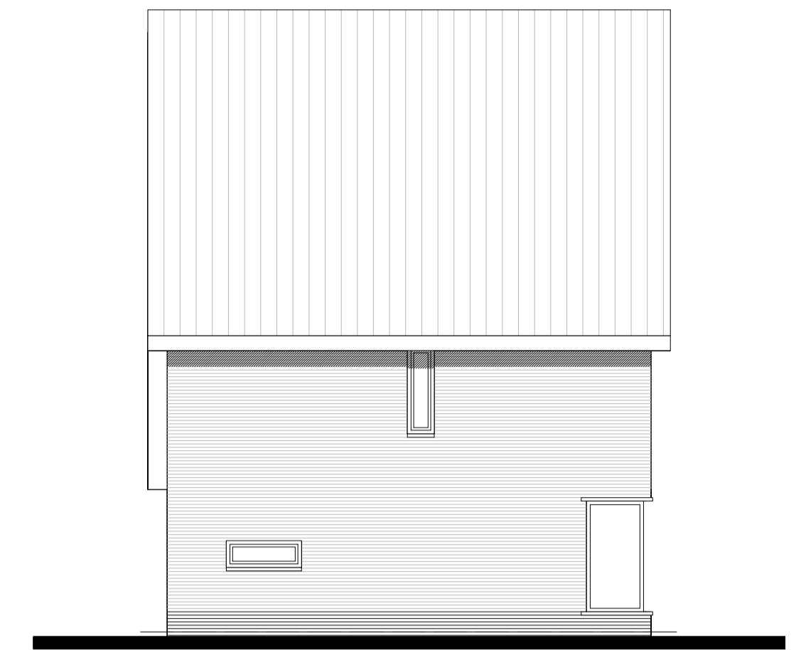
Linker aanzicht
