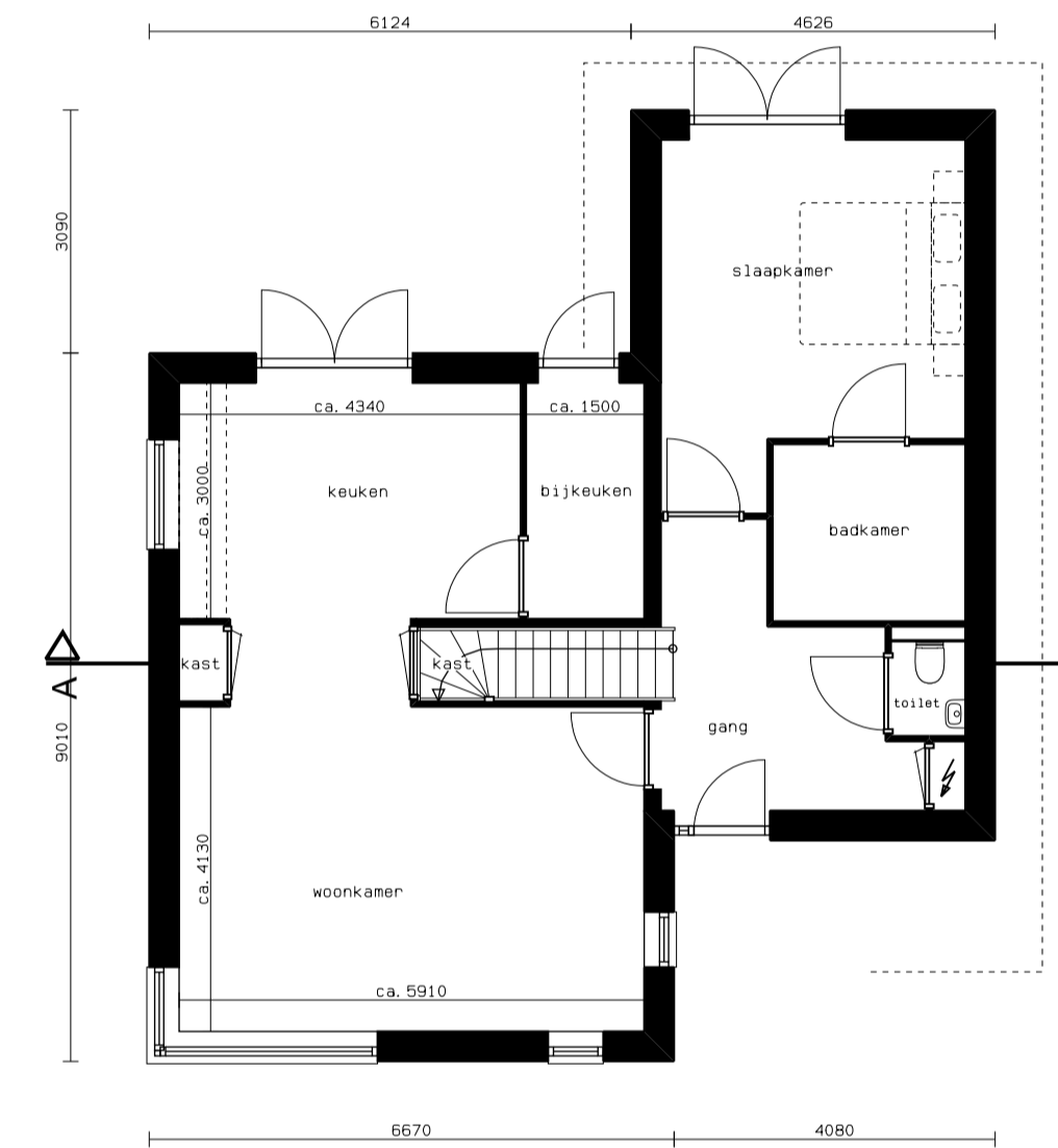
BEGANEGROUND 0.000+P (variant met slaapkamer)
